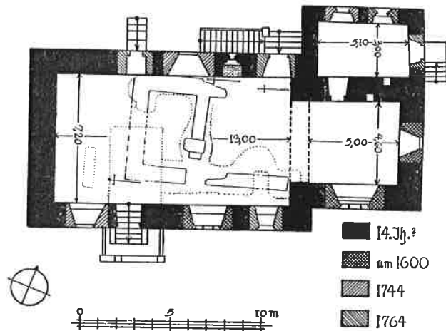
37. Kieselbronn. Pfarrkirche. Grundriß mit Grabungsergebnissen von 1935.
